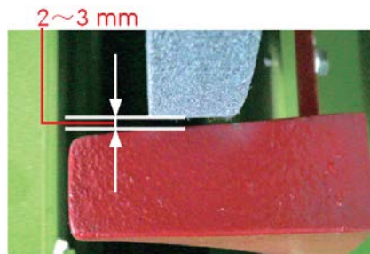
調整扶刀架間隙
